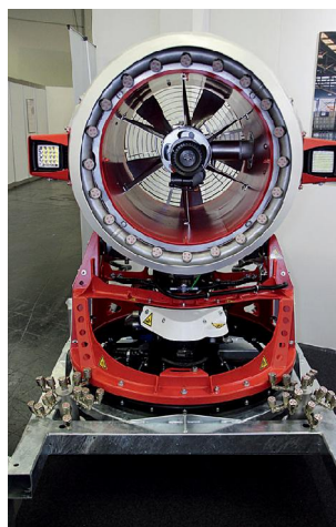
Löscherturbine: Emicontrols aus Bozen stellte eine stationäre Brandbekämpfungsturbine vor. Das Alleinstellungsmerkmal des Typs FT10e ist die Erzeugung und Abgabe von Wasserdampf zwischen 50 und 75 m. Auch Löschschaum kann erzeugt werden.
