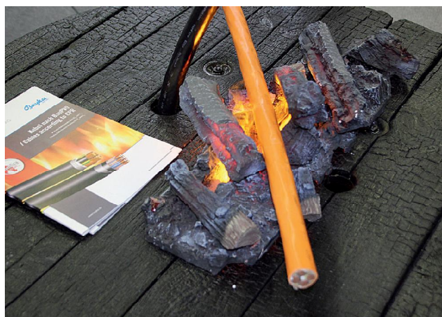
Bayerische Kabelwerke AG: Für Gebäude mit hohem Sicherheitsbedarf sowie generell für Fluchtwege empfehlen Experten der Branche die Brandschutzklasse B2ca. Die Kabelindustrie rät bereits seit Langem dazu, im vorbeugenden Brandschutz generell sogenannte Brandschutzkabel einzusetzen.
